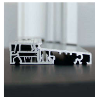
Seuil plat de 20 mm adapté PMR
